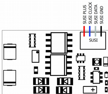
LD-G-33 plus mit PluX22-Schnittstelle - Rückseite -
