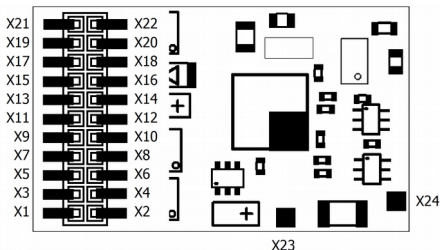
LD-G-33 plus mit PluX22-Schnittstelle - Vorderseite -
