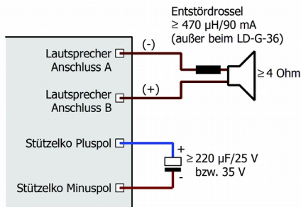
Fig. 4: Anschluss eines Stützkelkos zur Verbesserung der Spannungsversorgung und einer Entstördrossel am Lautsprecher
